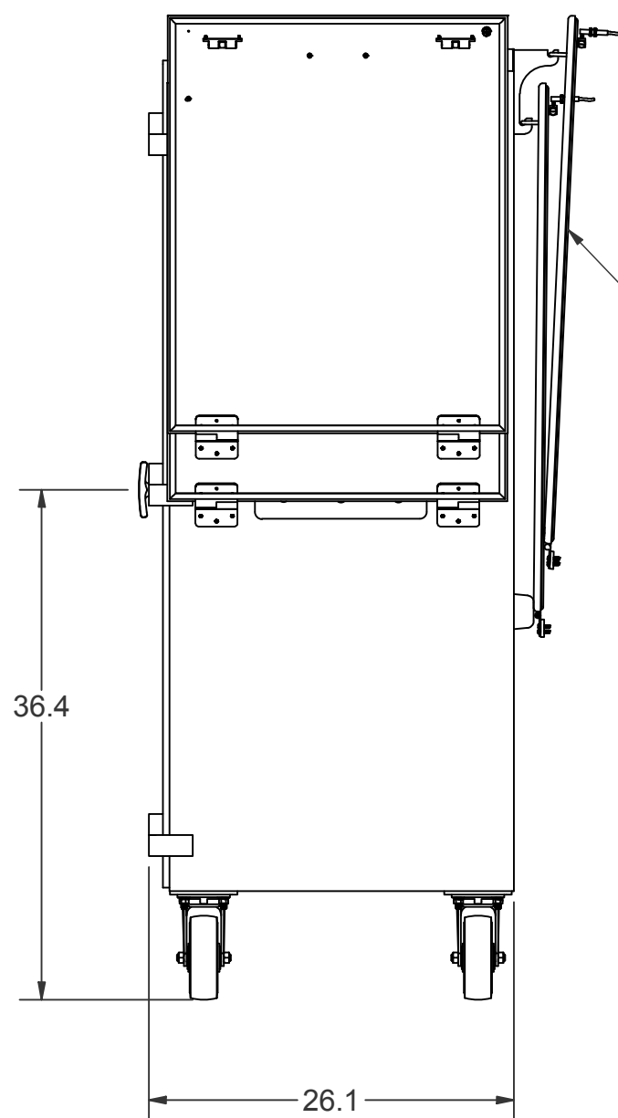
DOORS OPEN SCALE 0.08 : 1
